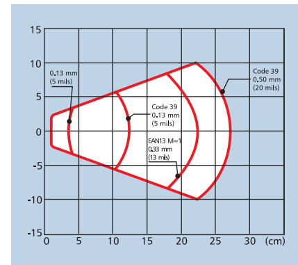
Area di lettura standard (10° skew angle)
